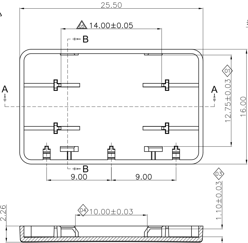
剖面 A-A
