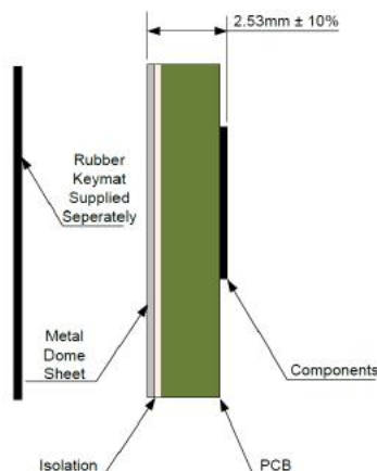
Figure 1.4: Stack-Up (D) - Thickness: PCB + isolation + metal dome sheet
